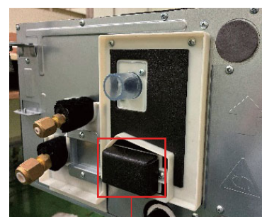
センサーケース
