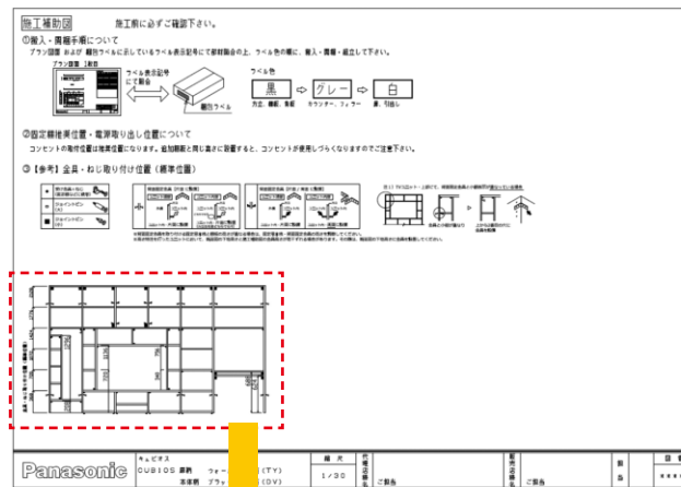
施工補助図
