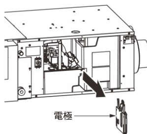
電極 FY-XEU350
